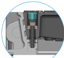
CHC locking
