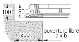
hauteur de cadre : 80 mm
