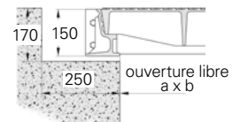
hauteur de cadre : 150 mm
